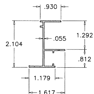
3A FRAME JAMB
