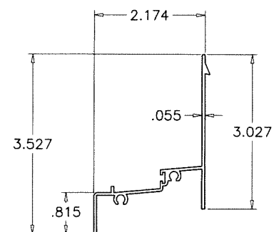
2A FRAME SILL
